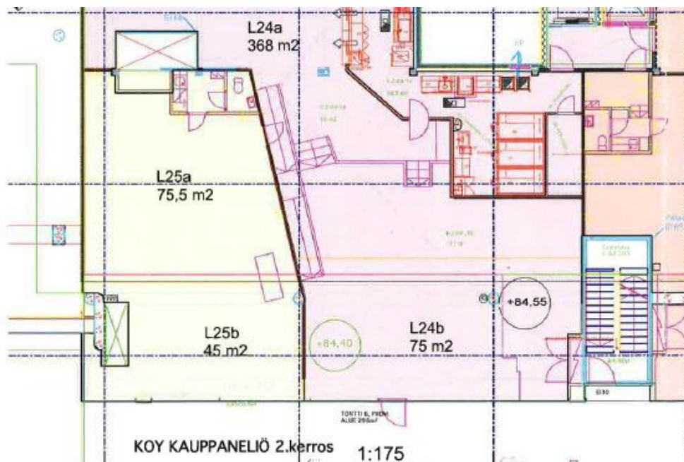
Liiketilan pohjakuva, L25a ja L25b.
